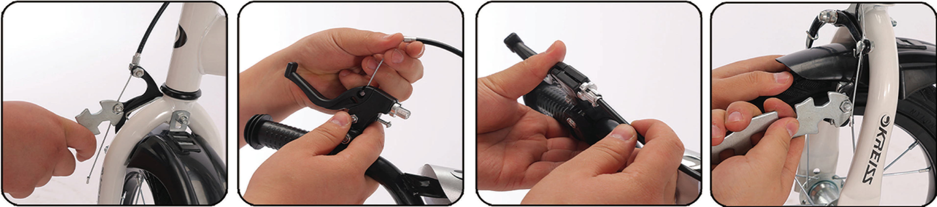
21. Ослабьте тормозные гайки. 22. Вытяните тормозной трос. 23. Проденьте трос в отверстие. 24. Ослабьте тормозные колодки. Отрегулируйте положение по горизонтали и затяните.
