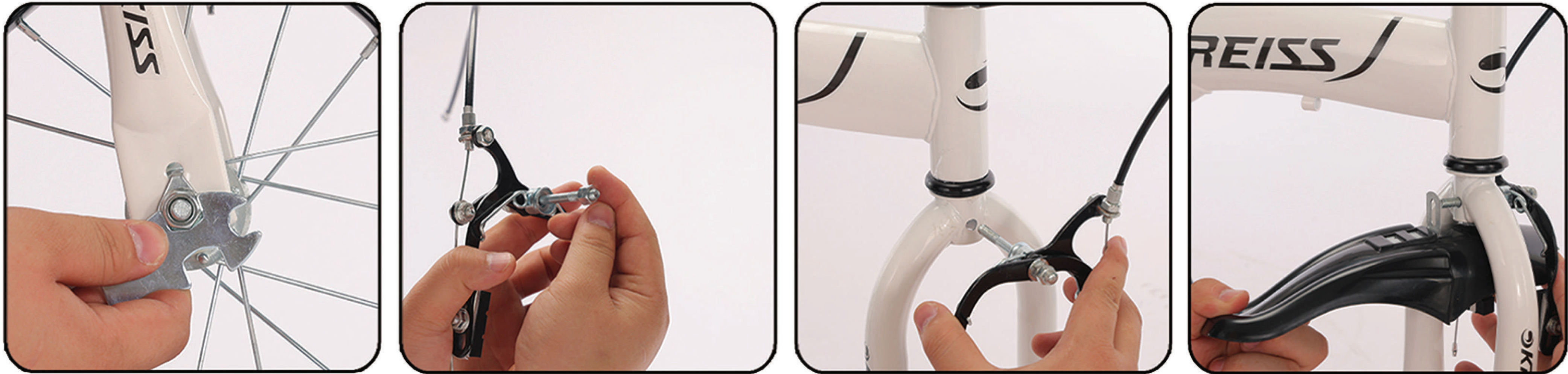
9. Прикрутите гайку обратно на переднее колесо и крепко затяните её. 10. Открутите винт на переднем тормозе. 11. Установите передний тормоз на переднюю вилку. 12. Короткое крыло должно быть спереди.
