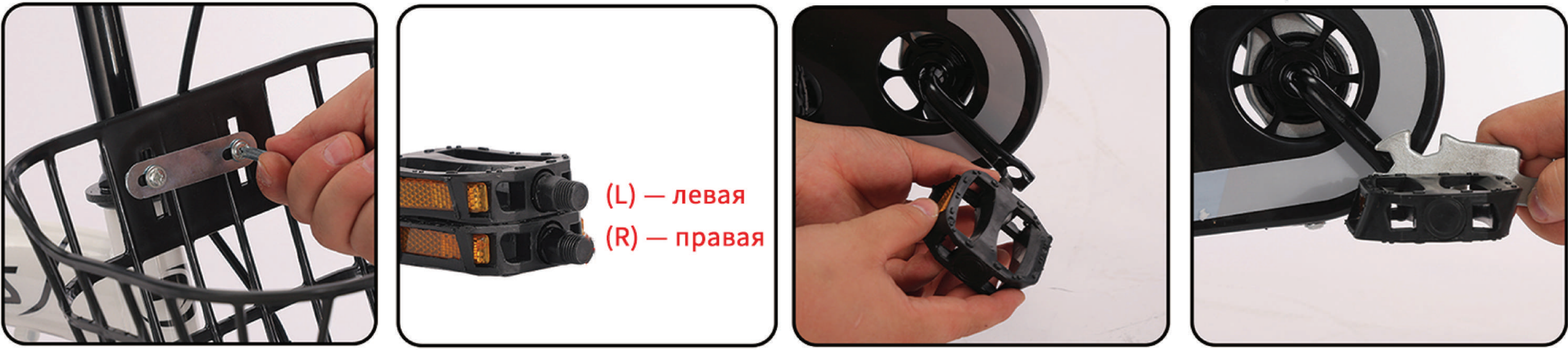
29. Закрепите корзинку на верхнем креплении. 30. Установите педали. 31. Закрутите правую педаль (R) по часовой стрелке, а левую педаль (L) - против часовой стрелки. 32. Затяните педали.
